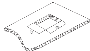
桌面安装方式开孔尺寸图 (单位：mm)
