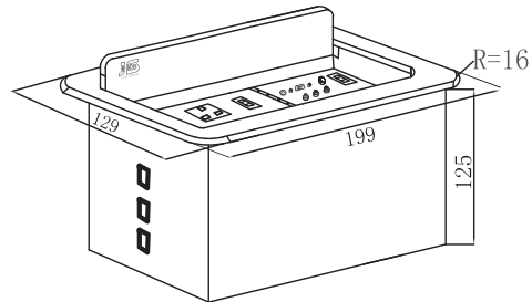
整体尺寸图 (单位: mm)
