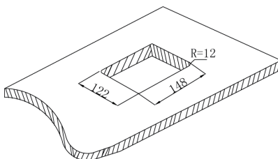
Cutout Dimension( mm)
